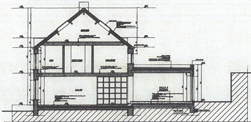
COUPE 1-1 PROJETEE
