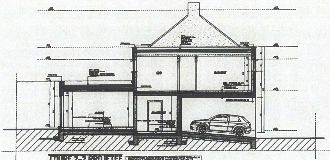
COUPE 2-2 PROJETEE
