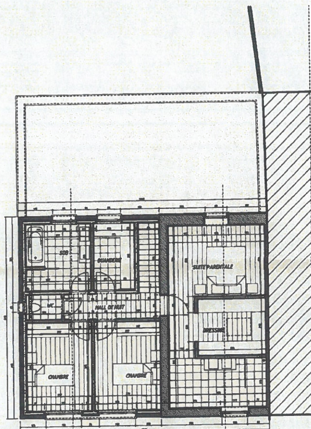
PREMIER ETAGE PROJETE
