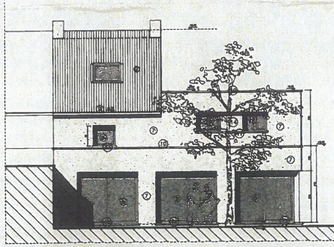
ELEVATION ARRIERE
