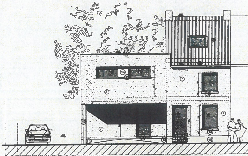
ELEVATION A RUE PROJETEE
