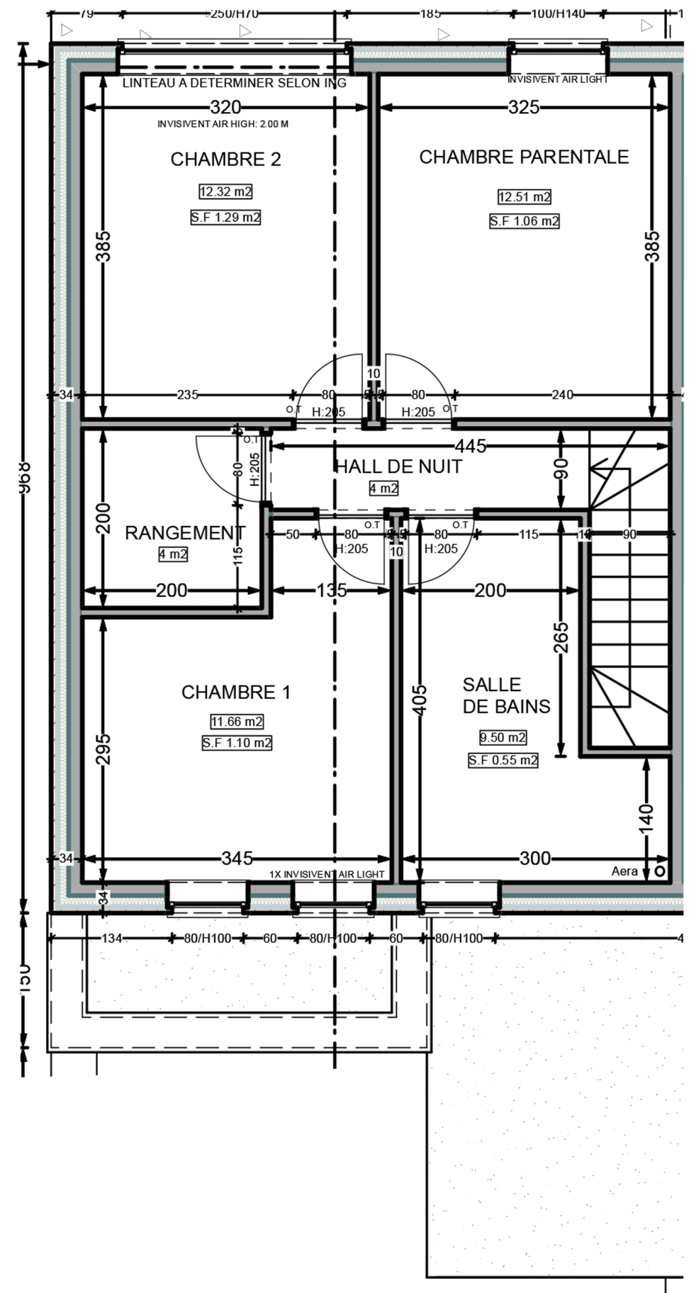
ÉTAGE
