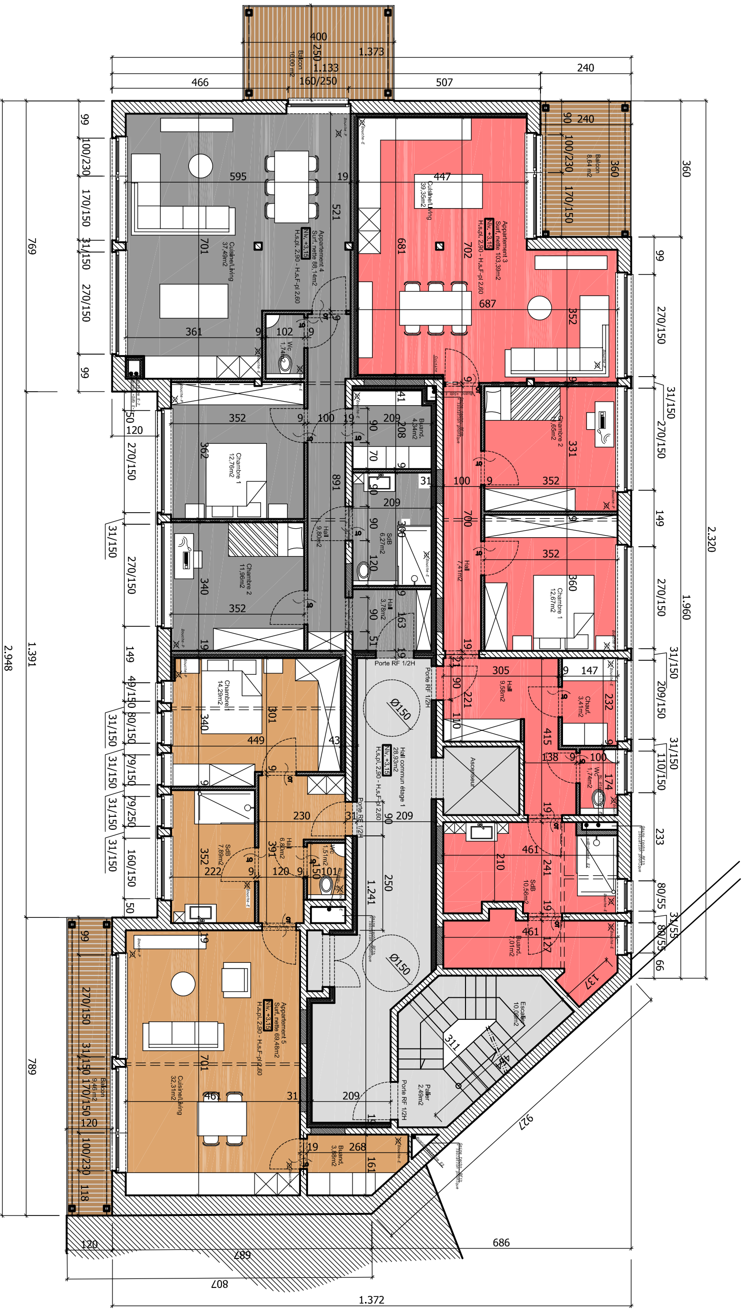
Vue en plan Etage 1 – Projeté Ech.: 1/100
