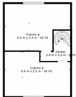
Étage 2
