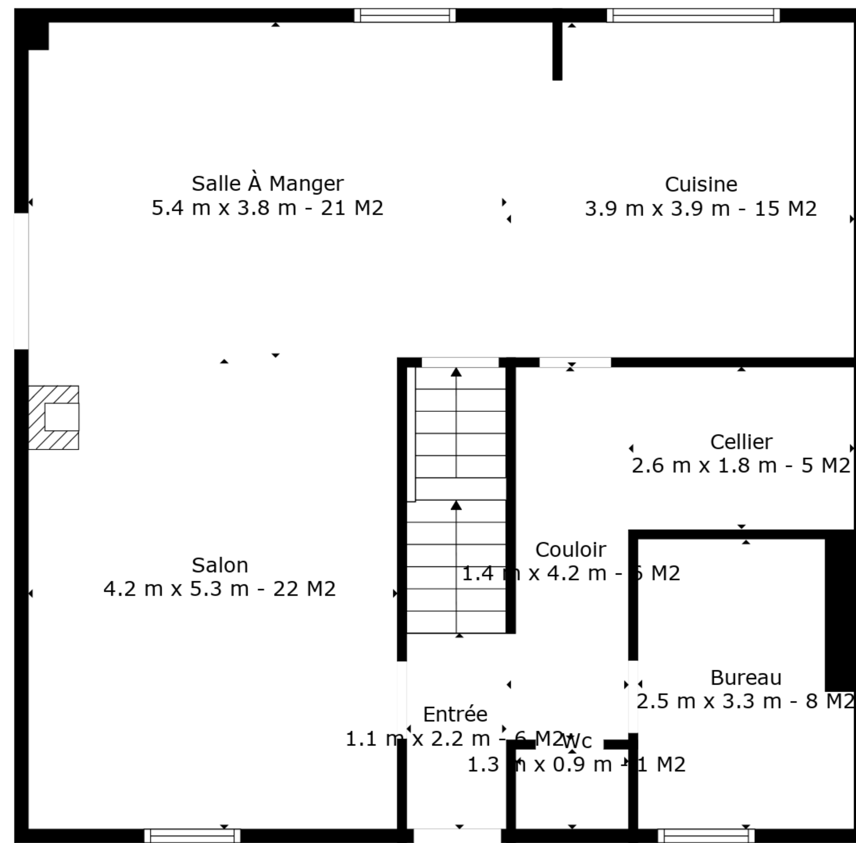
Étage 2
