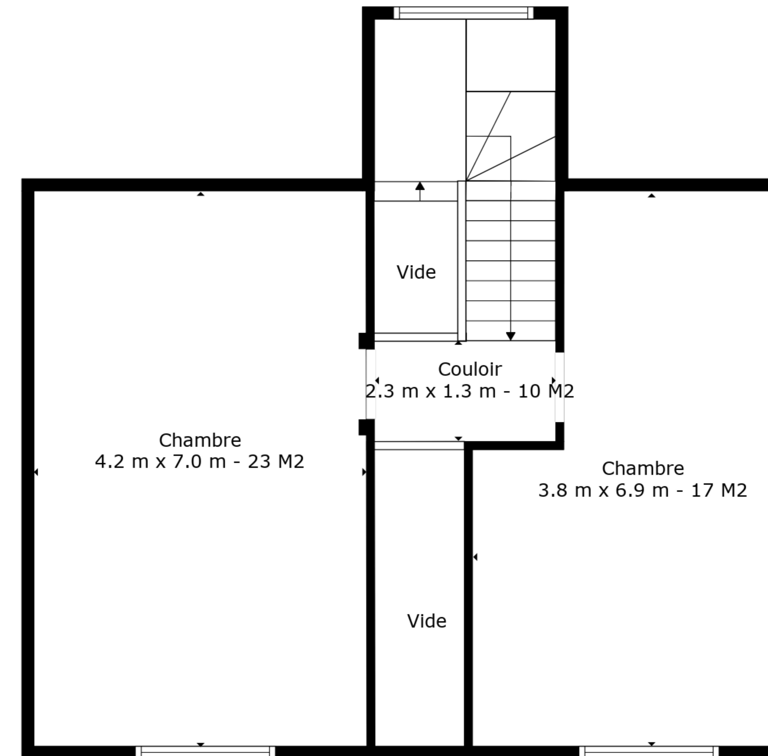
Étage 3
