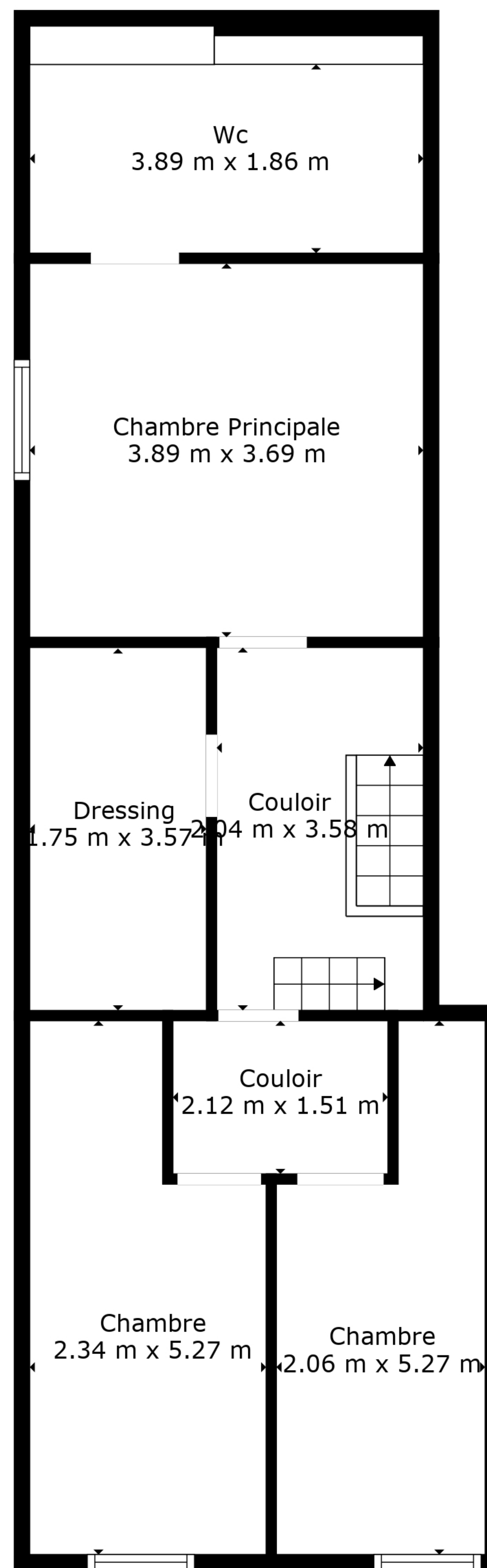
Étage 2
