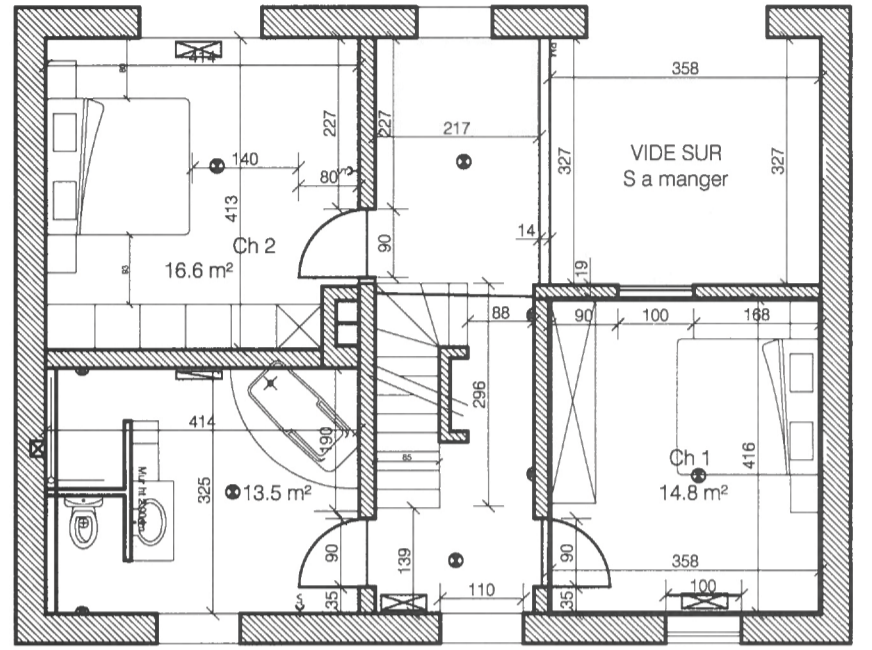
Etage 93 m 2
