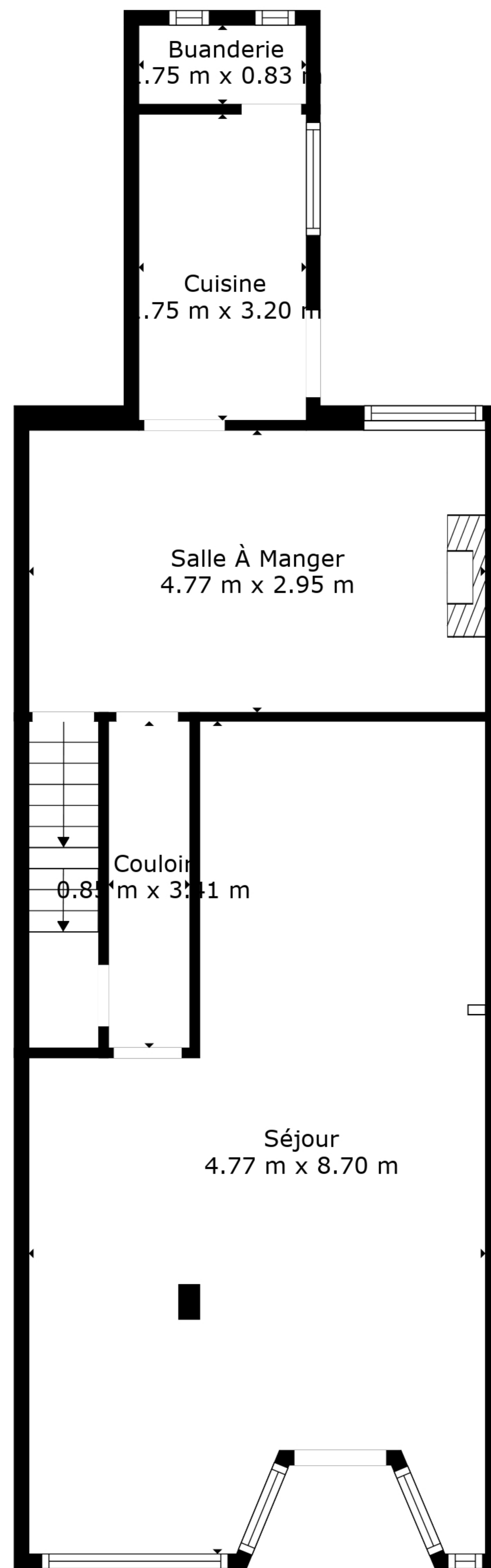
Étage 0
