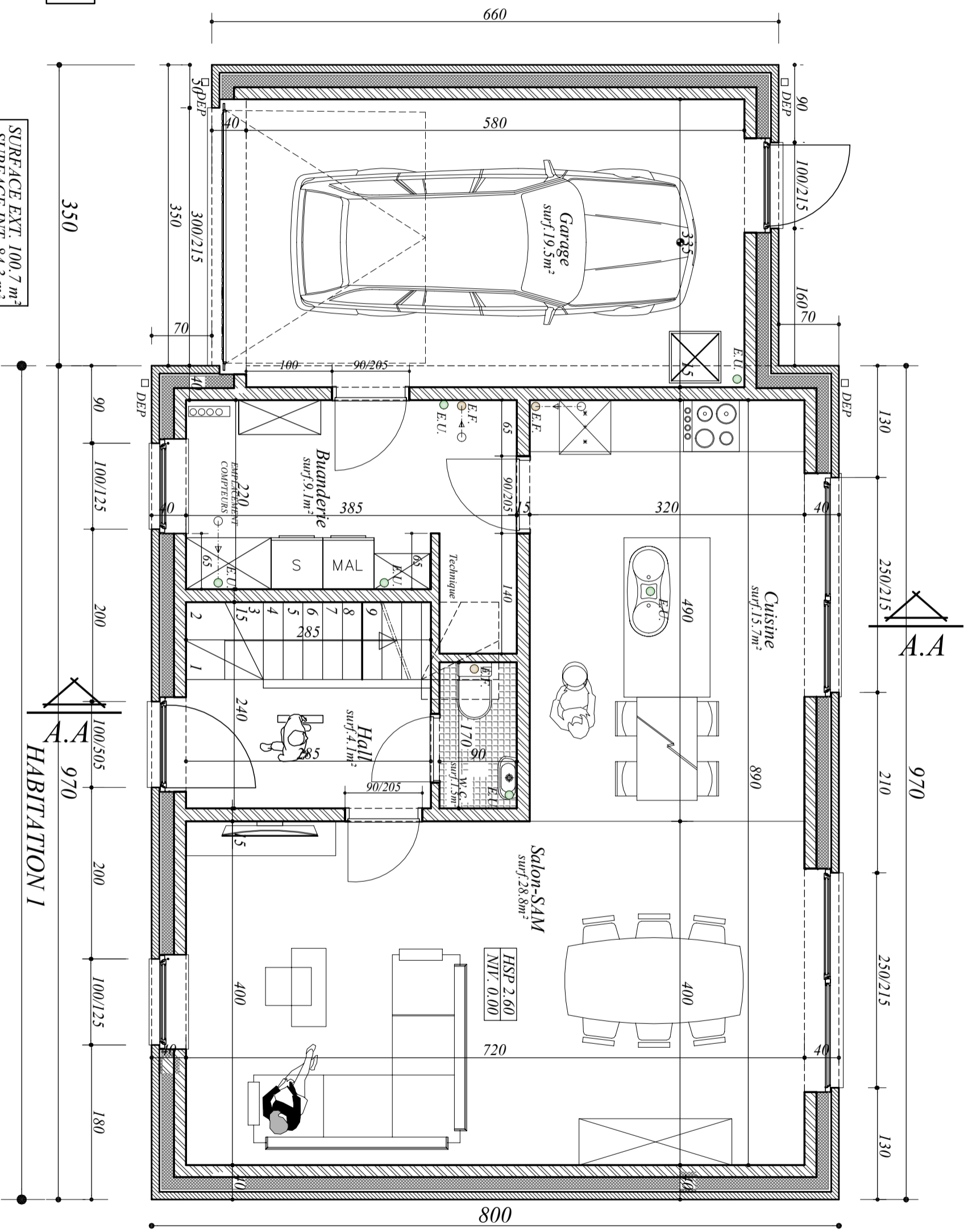
Plan du rez-de-chaussée éch. : 1/50e
