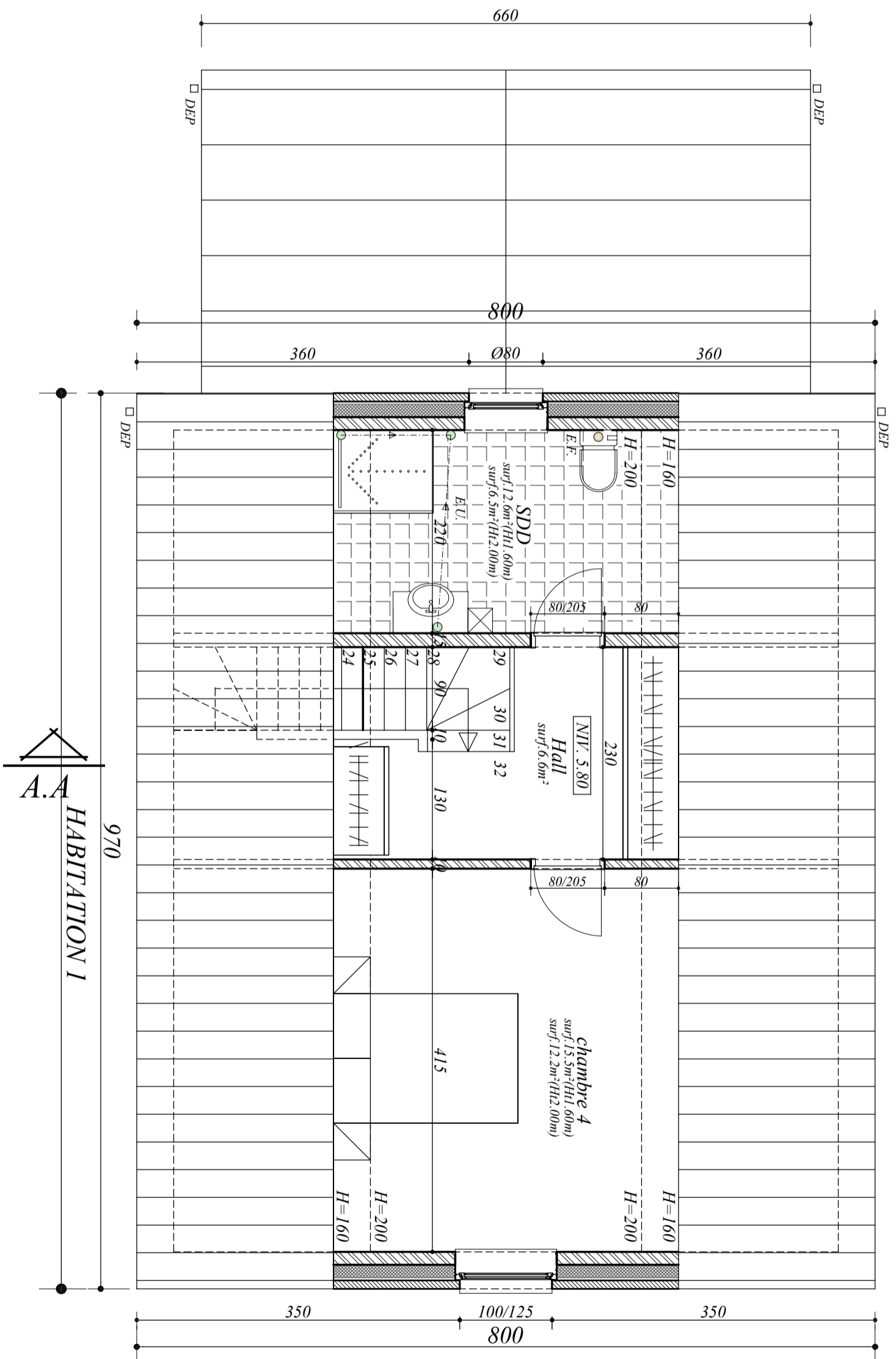
Plan des Combles éch. : 1/50e
